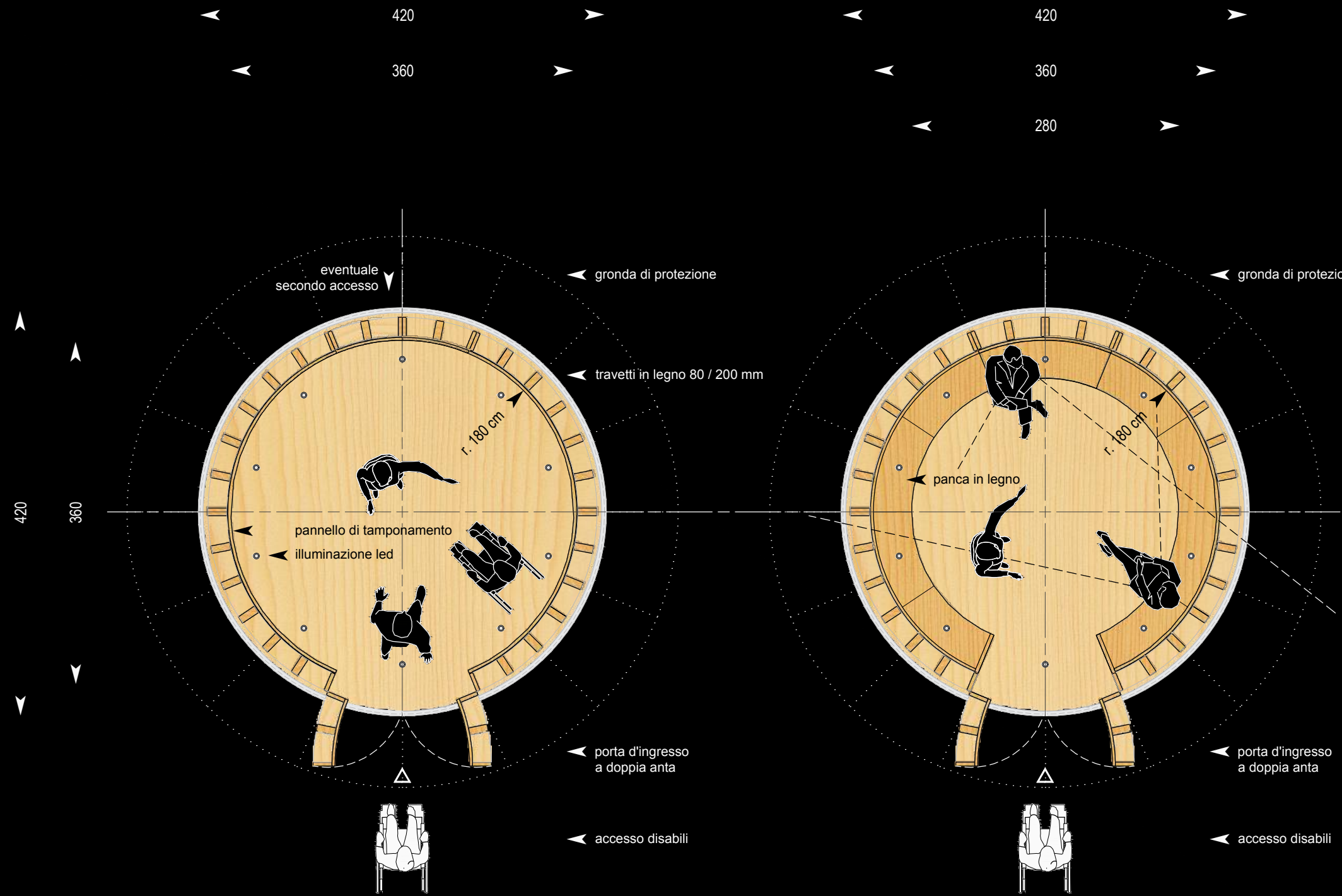
pianta 1 : 5 sezione + 1.00 pavillon senza arredamento e ingresso unico
